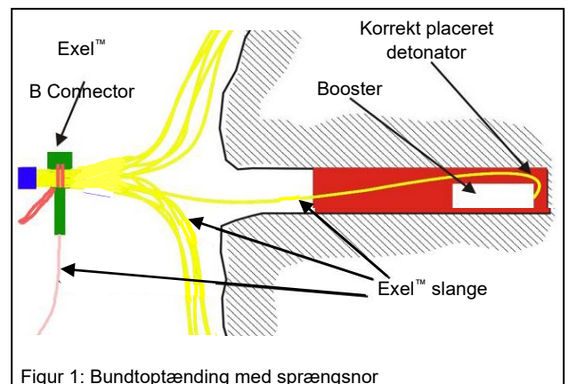
Figur 1: Bundtoptænding med sprængsnor
